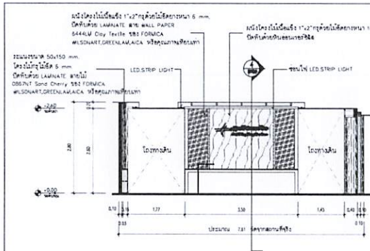
รูปด้าน 6 มาตราส่วน 1:75
