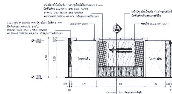
รูปด้าน 10 มาตราส่วน 1:75
