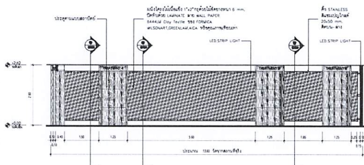
รูปด้าน 11 มาตราส่วน 1:75
