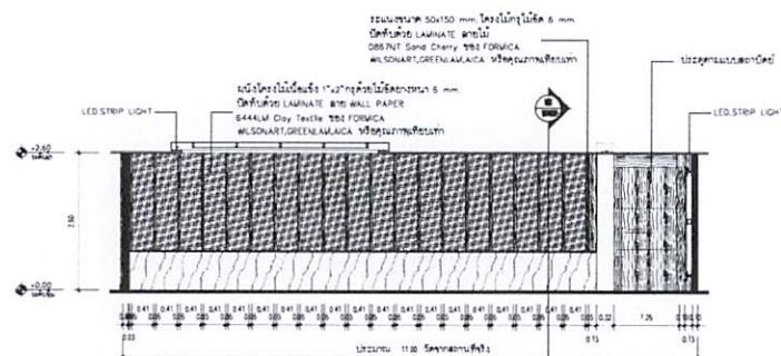
รูปด้าน 9 มาตราส่วน 1:75
