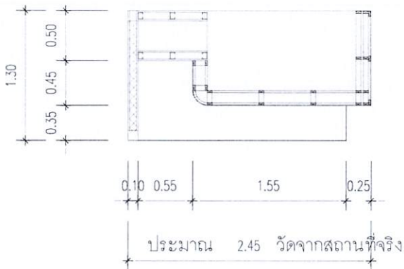
แปลน มาตราส่วน 1:25
