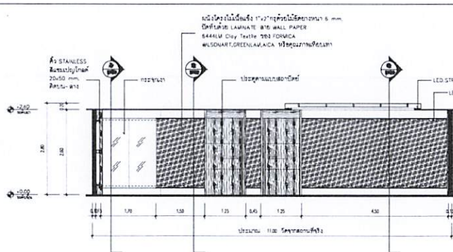
รูปด้าน 7 มาตราส่วน 1:75
