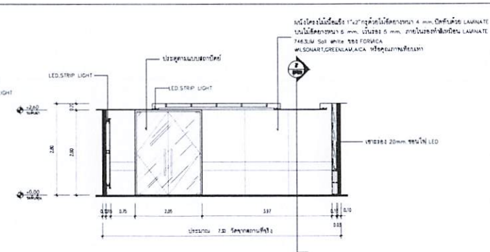
รูปด้าน 8 มาตราส่วน 1:75
