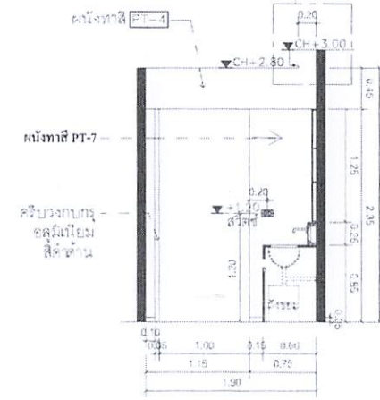
B ELEVATION 1:50
