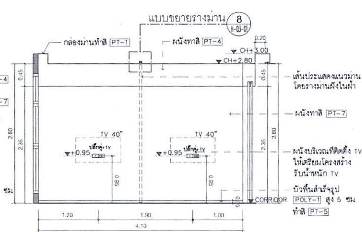
B ELEVATION 1:50 ห้องแปะยาชา 4
