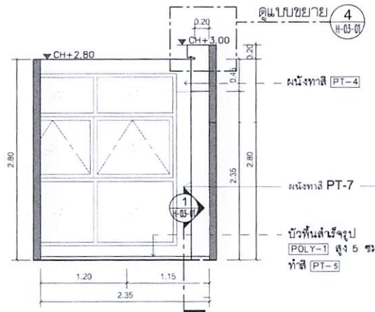
A ELEVATION 1:50 ห้องแปะยาชา 1
