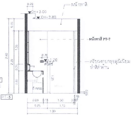
B ELEVATION 1:50 00-00-00
