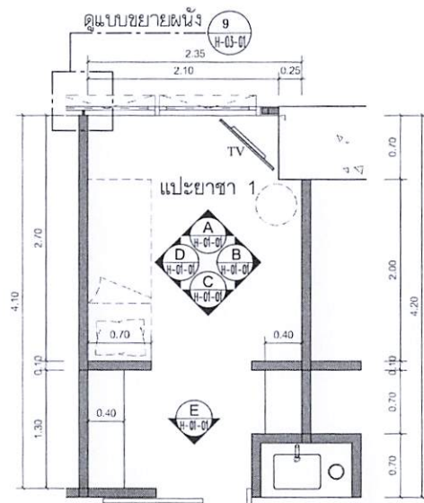
KEY PLAN 1:50 ห้องแปะยาชา 1
