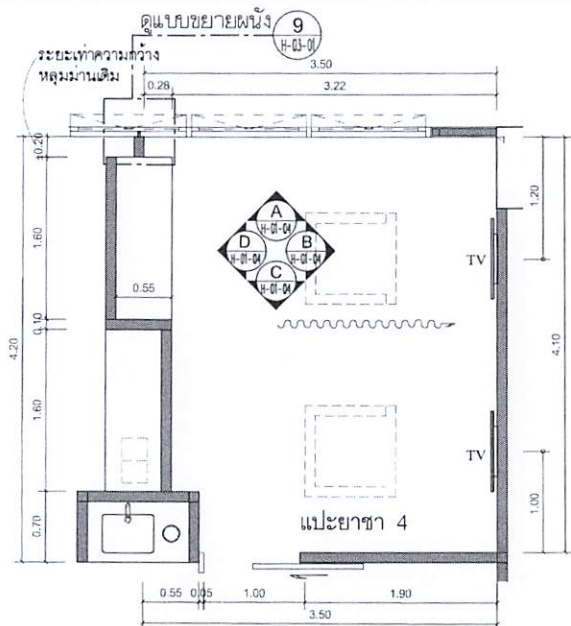
KEY PLAN 1:50 ห้องแปะยาชา 4
