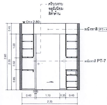
E ELEVATION 1:50 ห้องแปะยาชา 1
