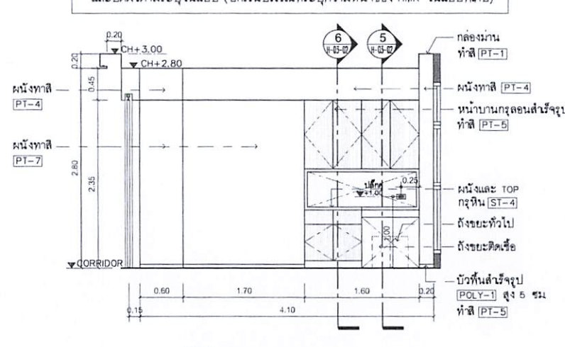
D ELEVATION 1:50 ห้องแปะยาชา 4
