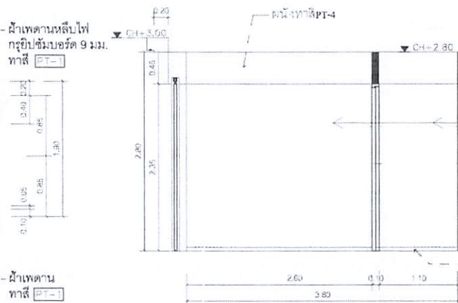
C ELEVATION 1:50 00-00-00
