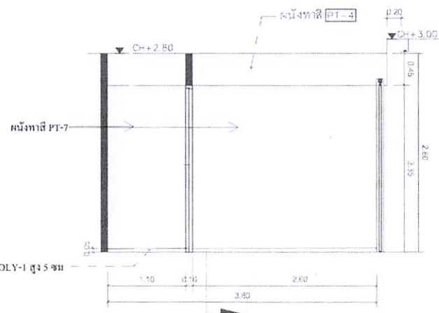
A ELEVATION 1:50 00-00-00
