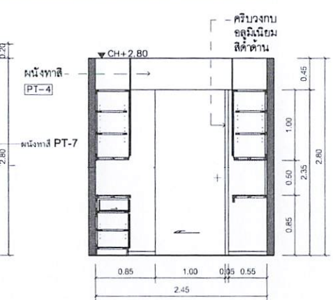
E ELEVATION 1:50 ห้องแปะยาชา 2
