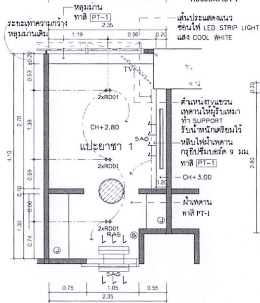
REFLECTED CEILING PLAN 1:50 ห้องแปะยาชา 1
