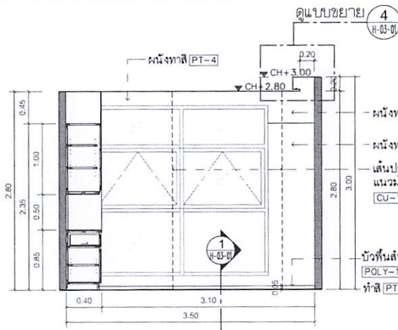
A ELEVATION 1:50 ห้องแปะยาชา 4
