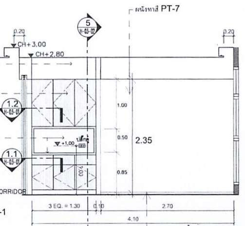
D ELEVATION 1:50 ห้องแปะยาชา 1
