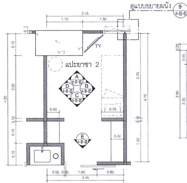
KEY PLAN 1:50 ห้องแปะยาชา 2
