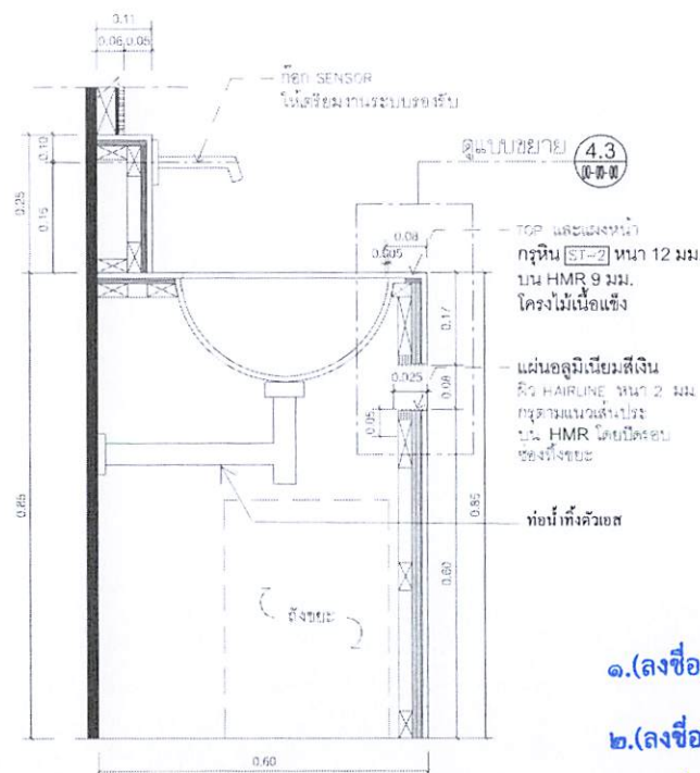
4.2 SECTION 1:10 (00-00-00)
