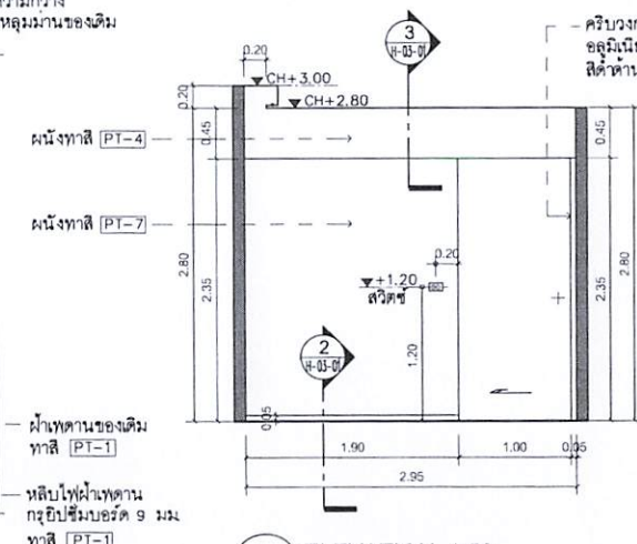
C ELEVATION 1:50 ห้องแปะยาชา 4
