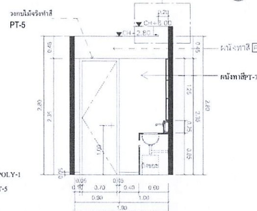
D ELEVATION 1:50 00-00-00
