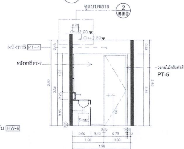
B ELEVATION 1:50
