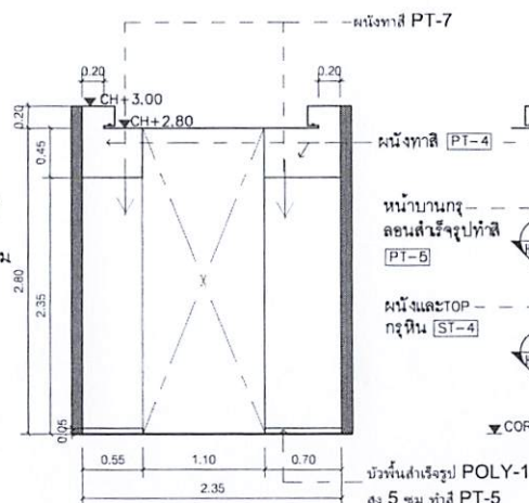
C ELEVATION 1:50 ห้องแปะยาชา 1
