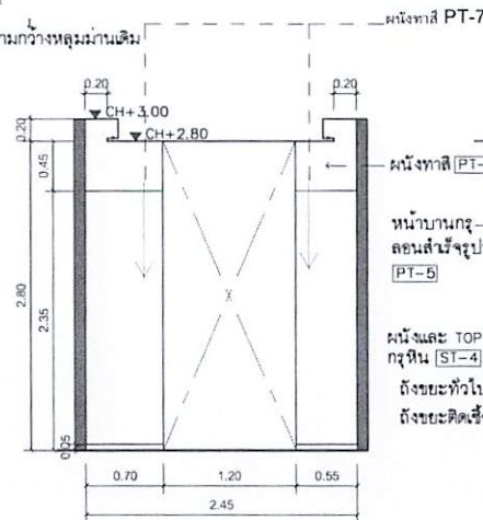
C ELEVATION 1:50 ห้องแปะยาชา 2
