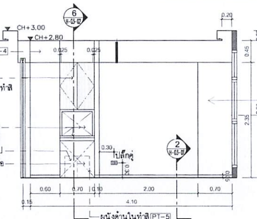
D ELEVATION 1:50 ห้องแปะยาชา 2
