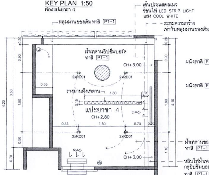
REFLECTED CEILING PLAN 1:50 ห้องแปะยาชา 4
