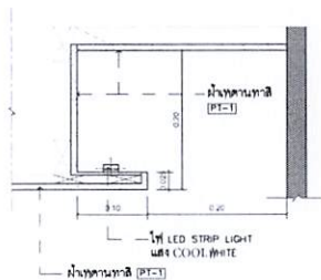
1 SECTION 1:5 ห้อง LASER B-9
