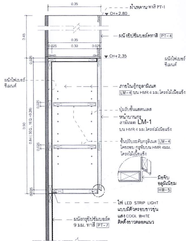
1 SECTION 1:10 ห้องชุดเชิ & ห้องเจาะเลือด
