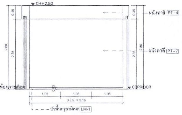
G ELEVATION 1:50 W-01-02 ห้องชุดเชื้อ & ห้องเจาะเลือด
