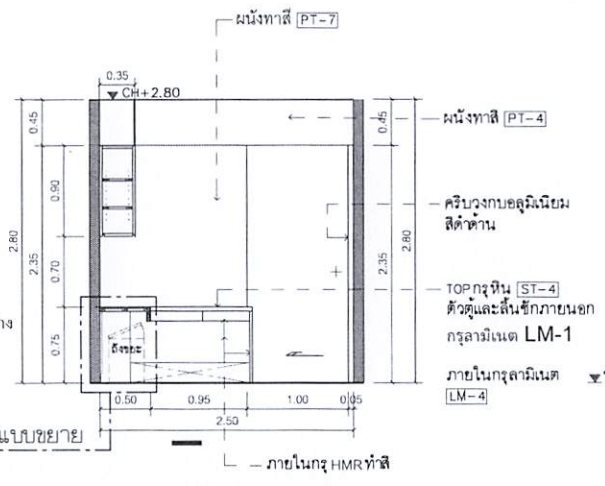
F ELEVATION 1:50 W-01-02 ห้องชุดเชื้อ & ห้องเจาะเลือด
