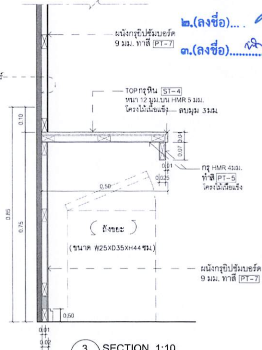
3 SECTION 1:10 ห้องชุดเชิ & ห้องเจาะเลือด
