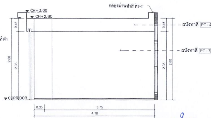
D ELEVATION 1:50 BODY 2
