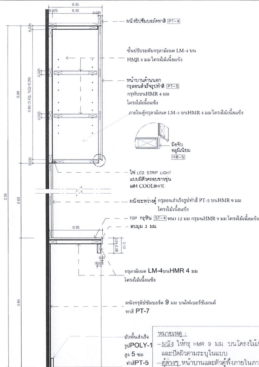
2 SECTION 1:10 ห้อง LASER B-9
