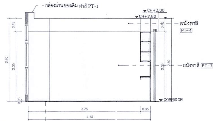
B ELEVATION 1:50 BODY 2
