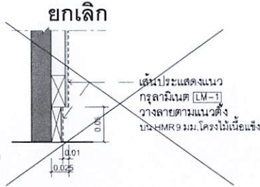
5 SECTION 1:5 ห้องชุดเชิ & ห้องเจาะเลือด
