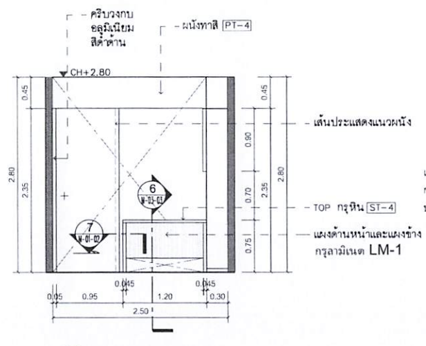
I ELEVATION 1:50 W-01-02 ห้องชุดเชื้อ & ห้องเจาะเลือด
