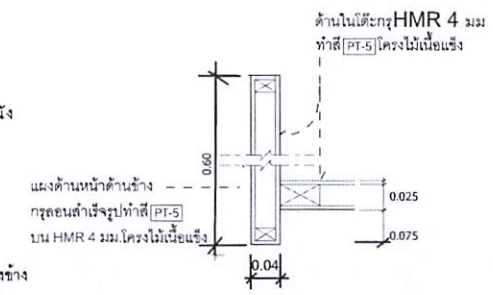
7 SECTION 1:5 W-01-02 ห้องชุดเชื้อ & ห้องเจาะเลือด
