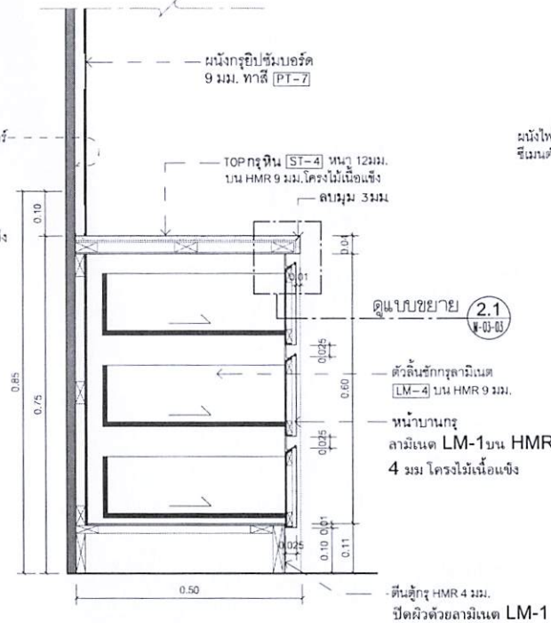
2 SECTION 1:10 ห้องชุดเชิ & ห้องเจาะเลือด
