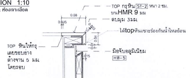
4.2 SECTION 1:5 W-03-02 ห้องชุดเอื้อ & ห้องเจาะเลือด
