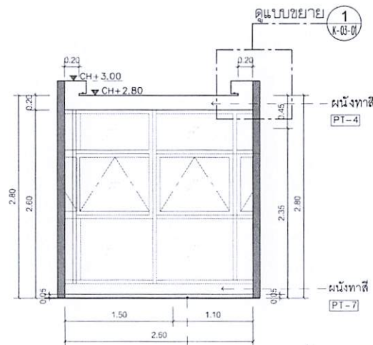
A ELEVATION 1:50 BODY 2
