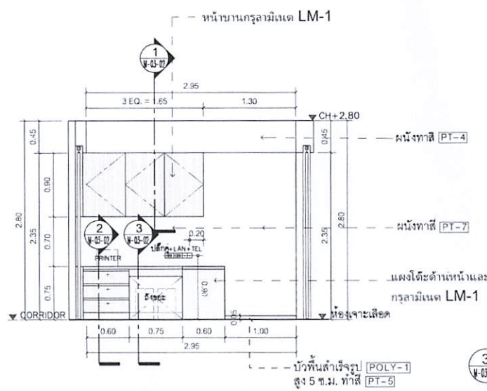
E ELEVATION 1:50 W-01-02 ห้องชุดเชื้อ & ห้องเจาะเลือด
