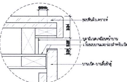
แบบขยาย A2 มาตราส่วน 1:2
