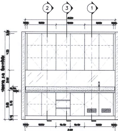
รูปด้านหน้า BF4.3 มาตราส่วน 1 : 25
