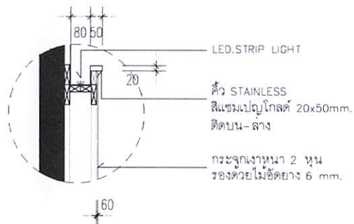
แบบขยาย 7 มาตราส่วน 1:10
