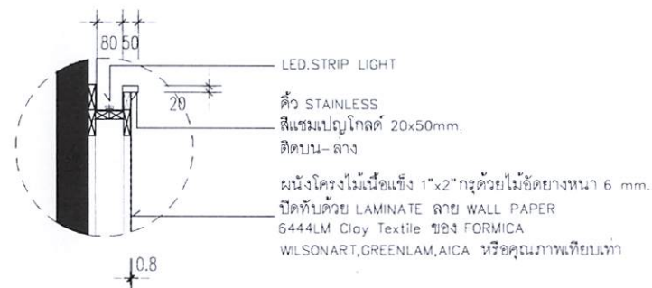
แบบขยาย 8 มาตราส่วน 1:10
