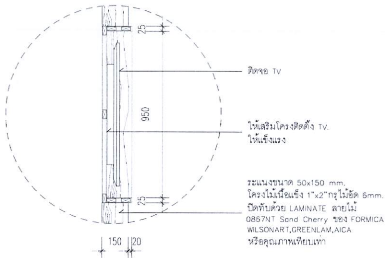
แบบขยาย 5 มาตราส่วน 1:10
