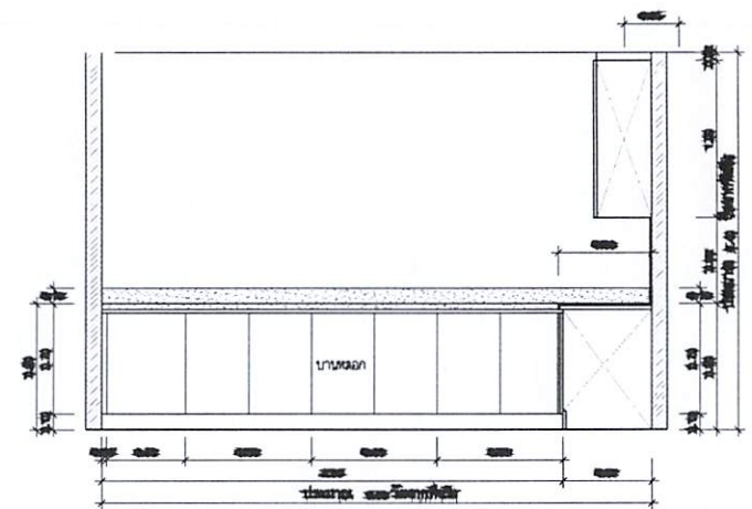
รูปด้าน BF4.4 B มาตราส่วน 1 : 25
