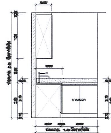
รูปด้าน BF4.4 C มาตราส่วน 1 : 25
